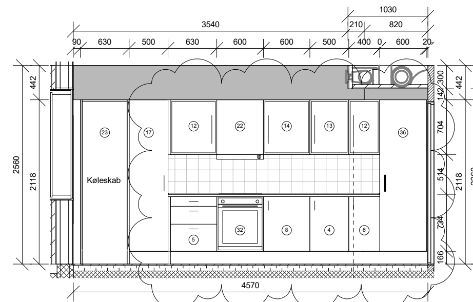
Snit C-C
