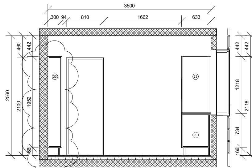
Snit A-A
