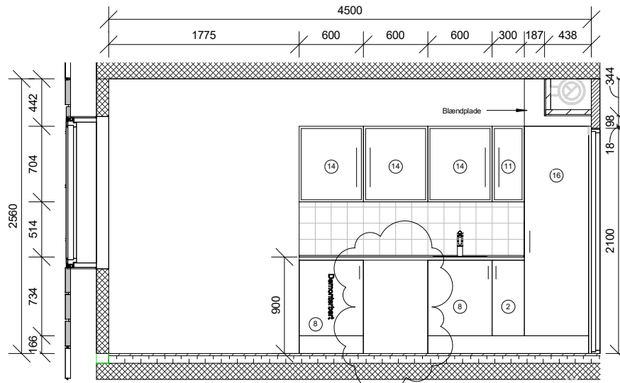
Snit A-A
