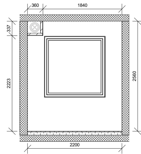
Snit C-C
