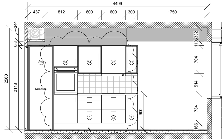
Snit C-C
