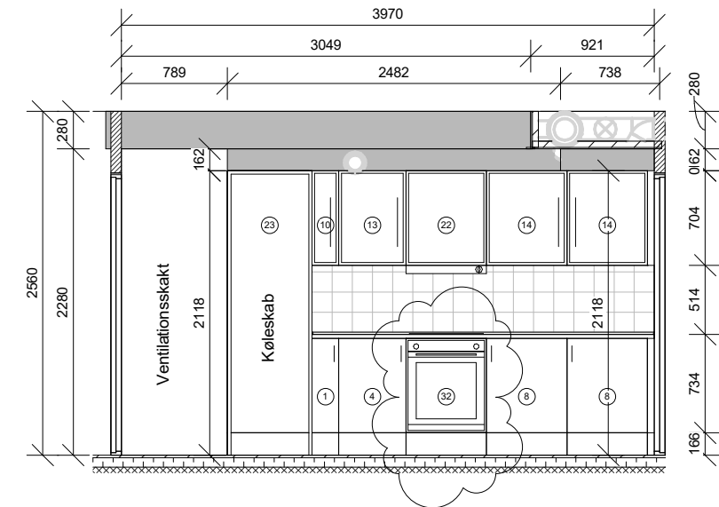
Snit D-D
