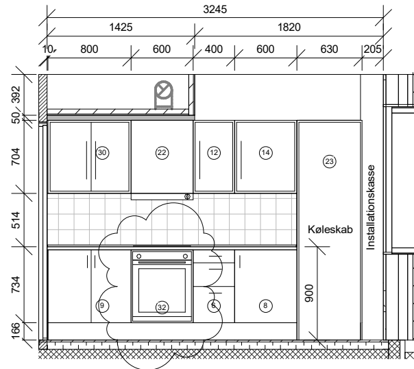
Snit A-A
