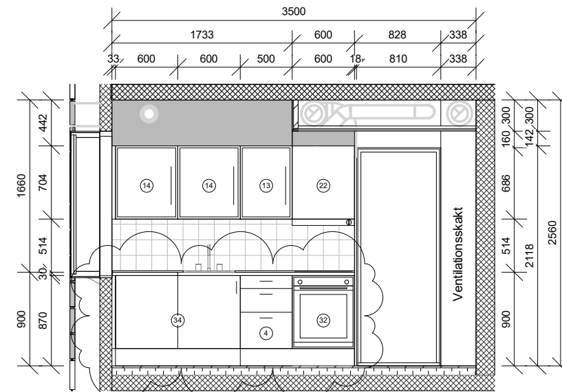
Snit D-D
