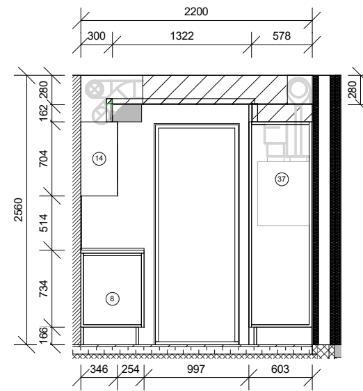
Snit A-A
