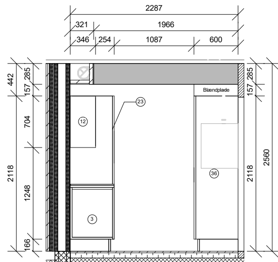
Snit C-C
