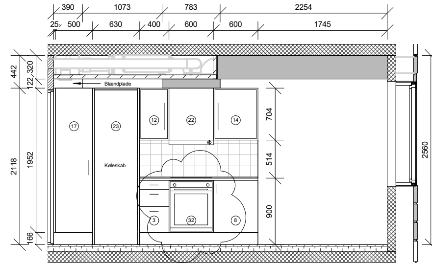
Snit A-A
