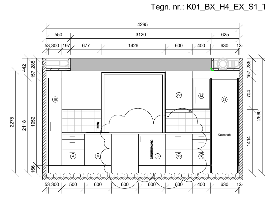
Snit B-B
