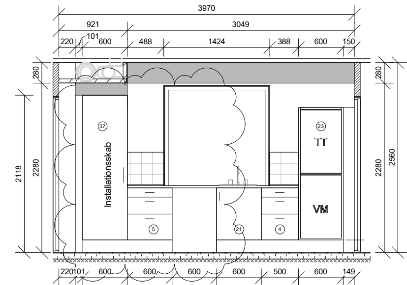
Snit B-B
