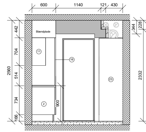
Snit B-B
