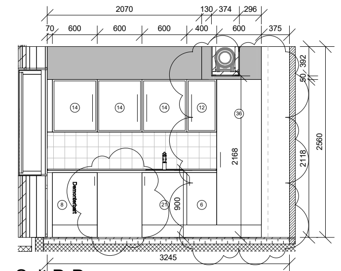
Snit D-D
