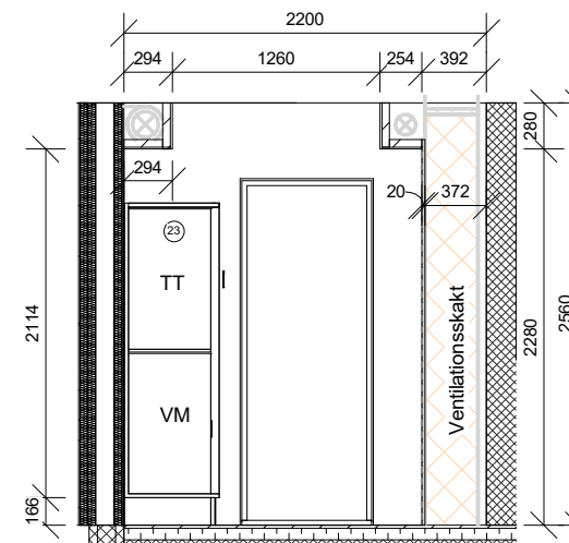
Snit A-A
