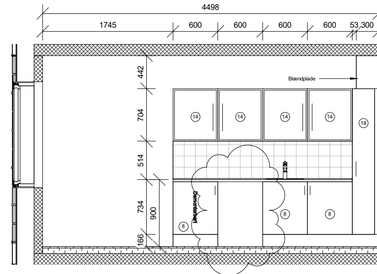
Snit C-C
