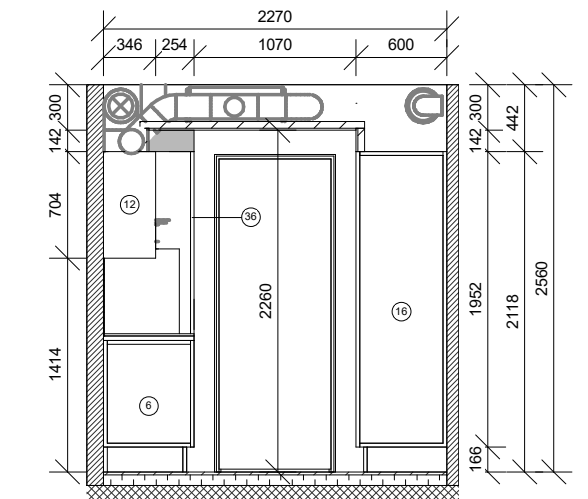
Snit D-D
