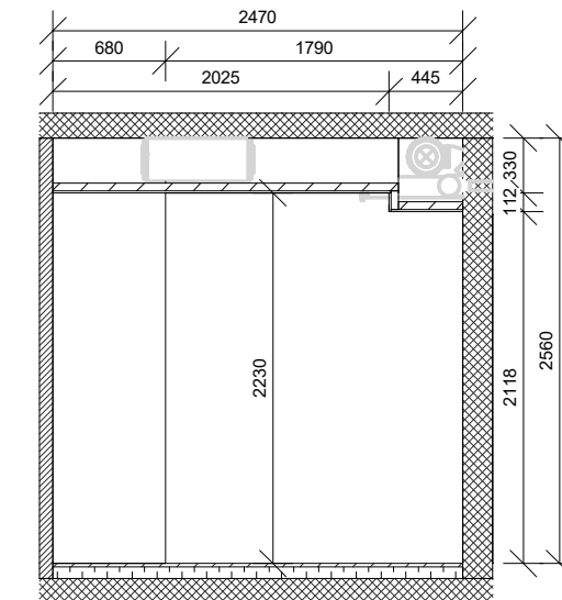
Snit D-D
