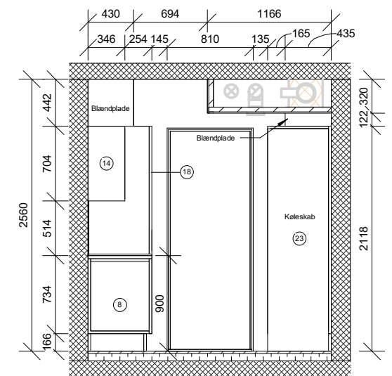
Snit D-D
