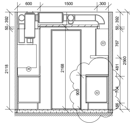
Snit A-A
