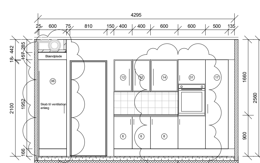
Snit D-D
