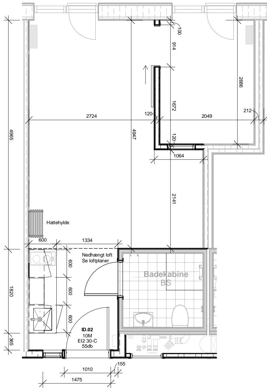
Boligtype B2R
