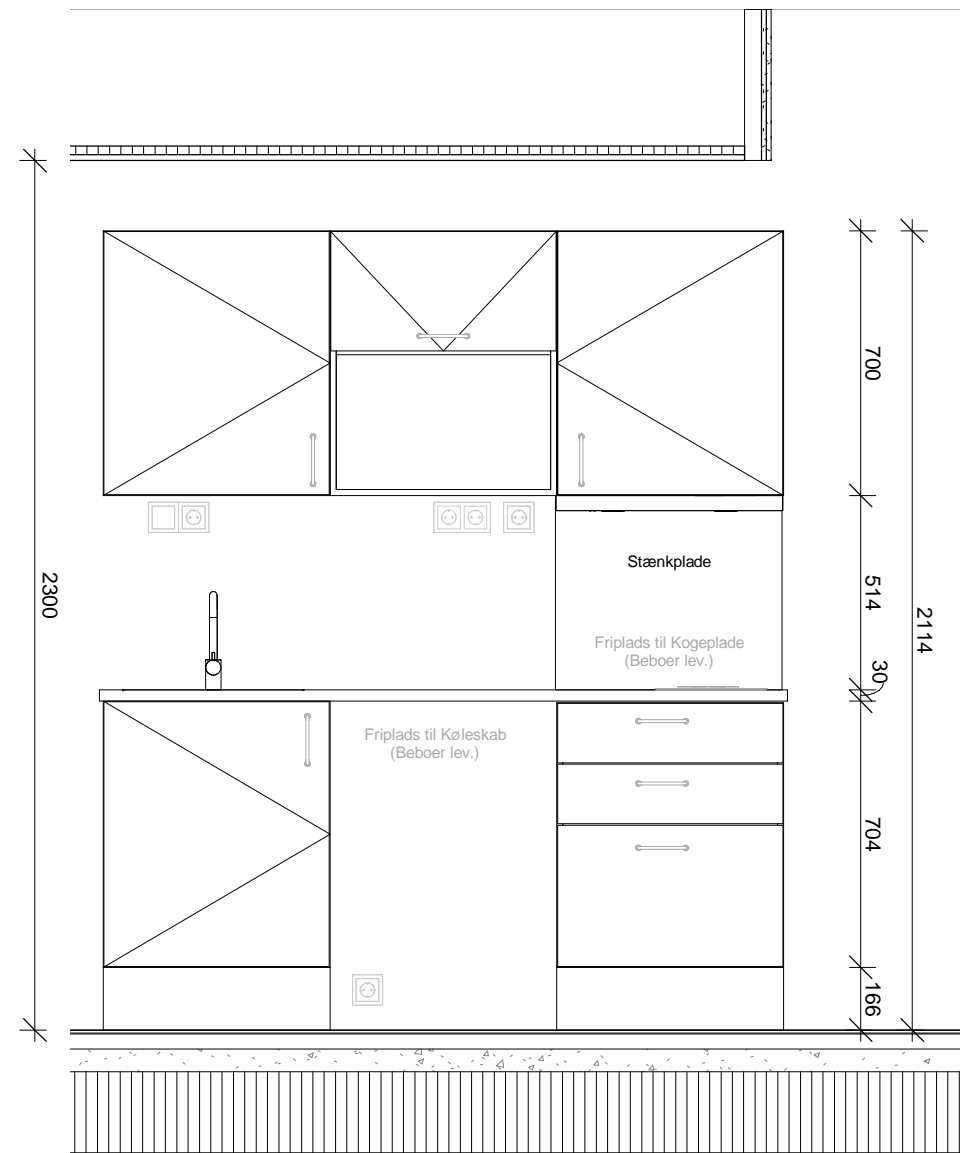
BV - Køkken - Opstalt 1 : 20
