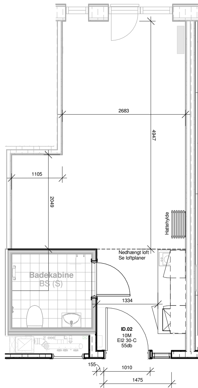
Boligtype BB 1 : 50
