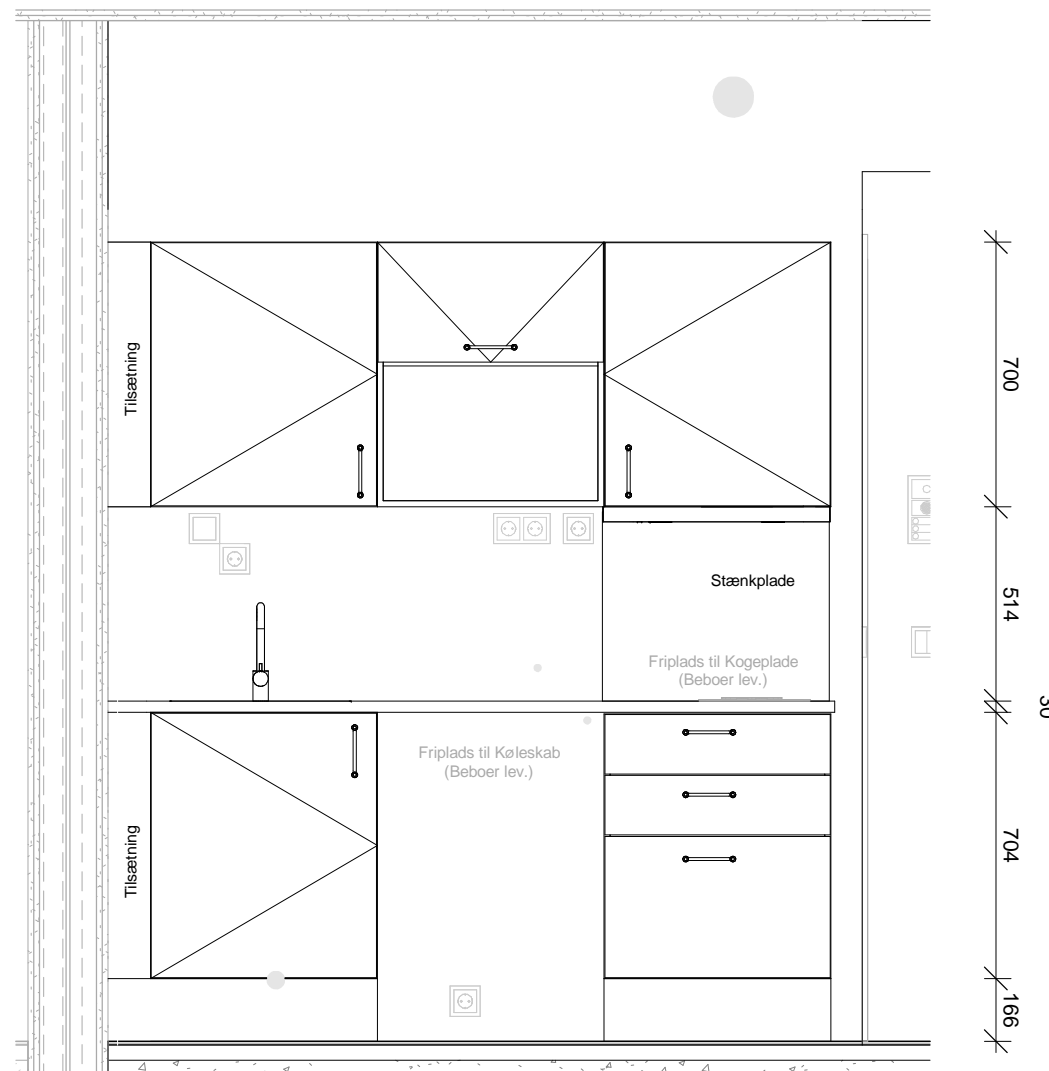
ABT - Køkkenopstalt 1 : 20
