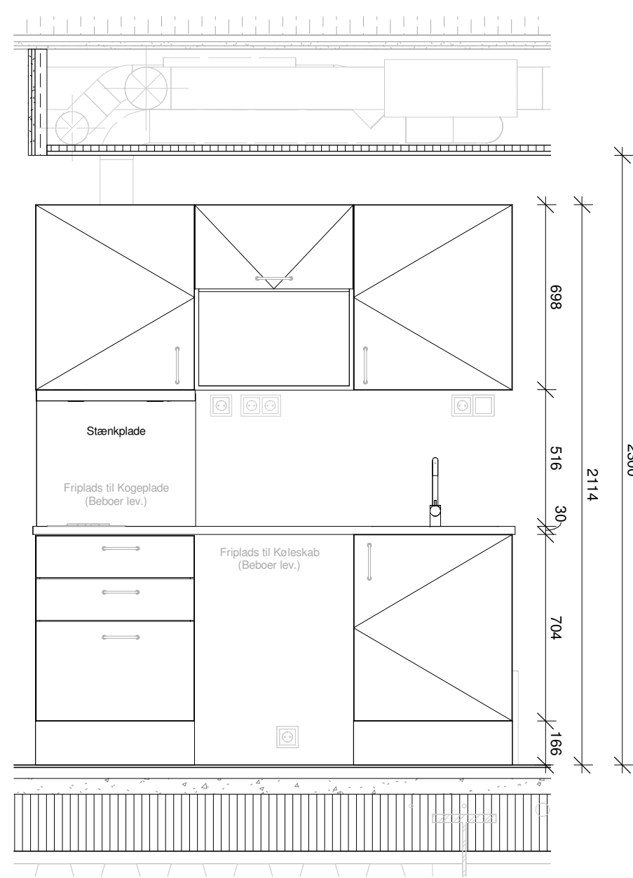
BB - Køkken Opstalt 1 : 20
