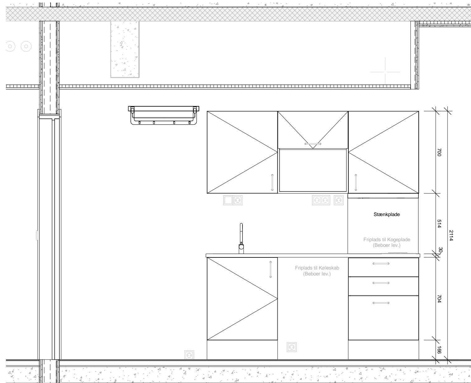
BS2 - Køkken - Opstalt 1 : 20
