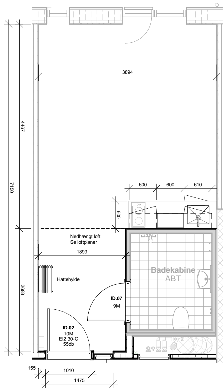
Bolitgtype ABT 1 : 50
