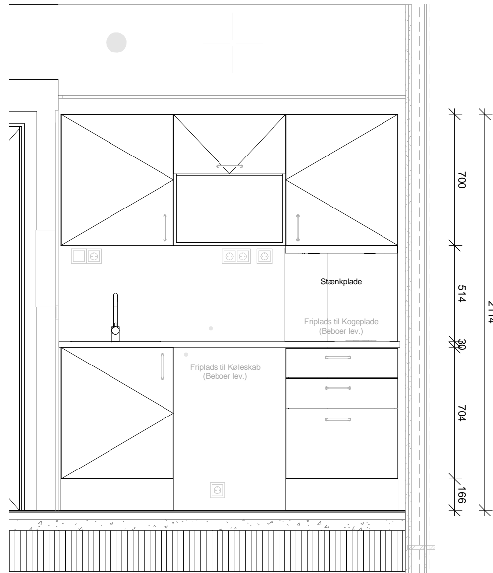
BS - Køkken - Opstalt 1 : 20
