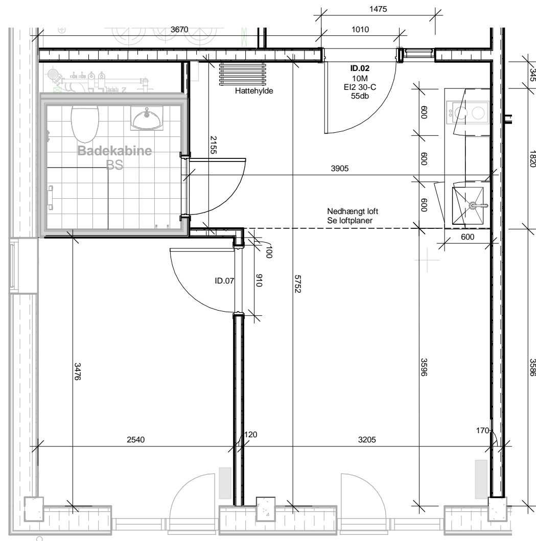
Boligtype B2RH 1 : 50
