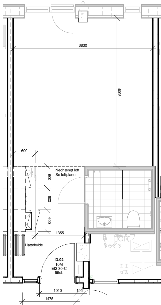
Boligtype BS2 1 : 50
