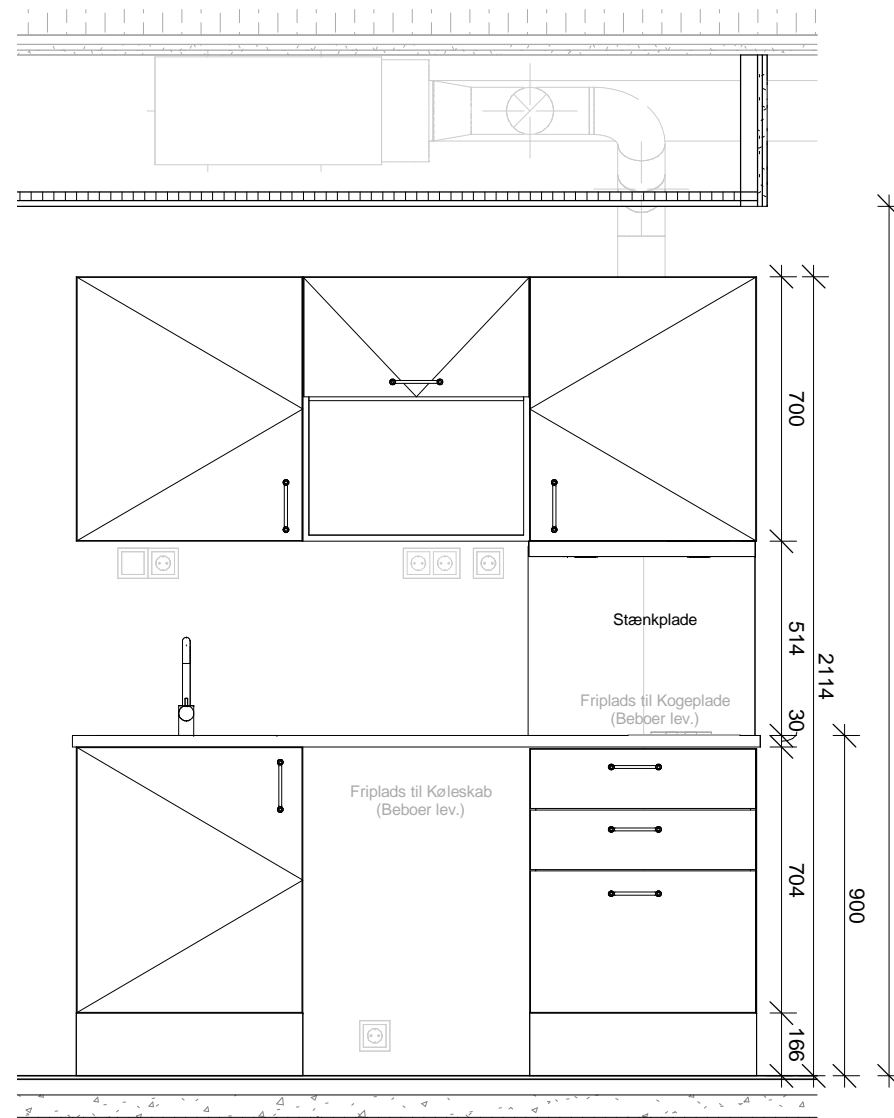
B2R - Køkken opstalt
