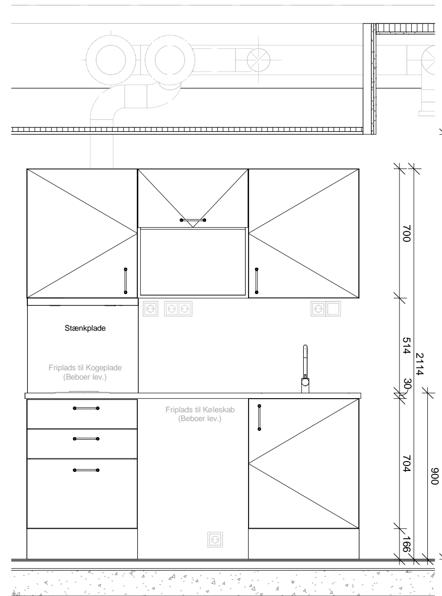
B2RH - Køkken opstalt 1 : 20
