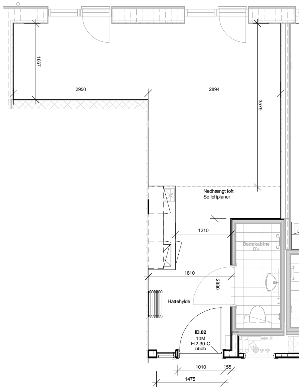
Boligtype BV 1 : 50
